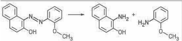
Μερικά από τα διαζωχρώματα τα οποία χρησιμοποιούνται στα τατουάζ, όπως το Solvent Red 1 (αριστερά), διασπώνται παράγοντας ενώσεις (δεξιά) που είναι ουσίες, οι οποίες ενδεχομένως είναι καρκινογόνες [Chemicaland Engineering News, Aug., 2016].
